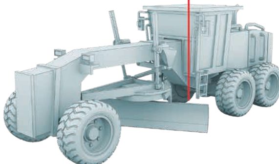
Konfiguracija s dvostrukim laserskim prijamnikom
